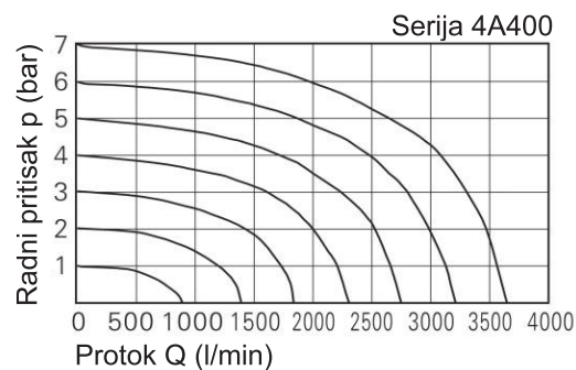
Dijagram protoka
